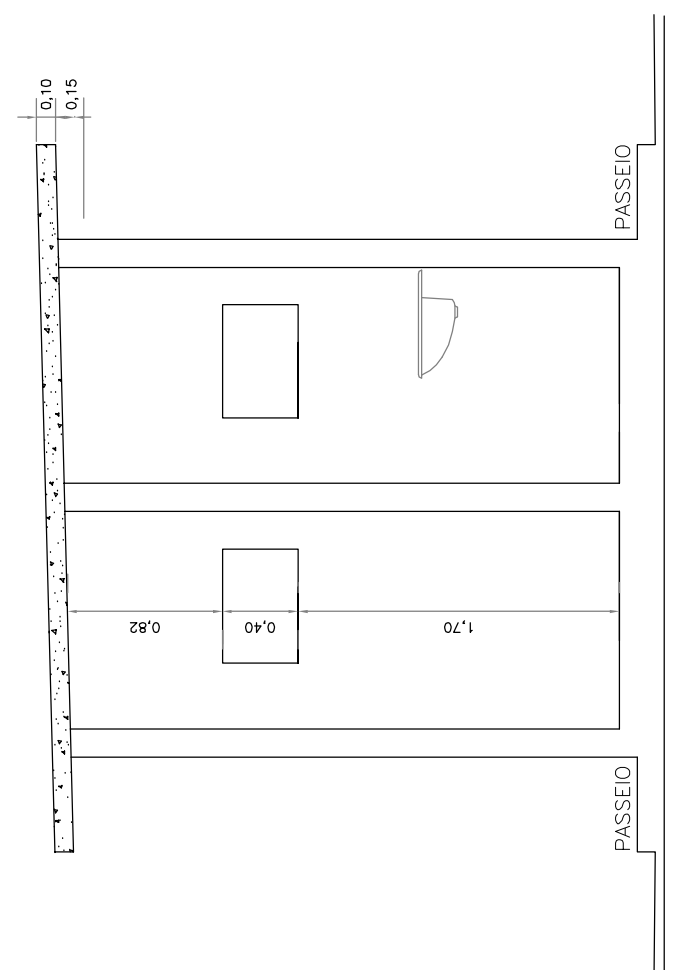
CORTE BB ESCALA 1:40
